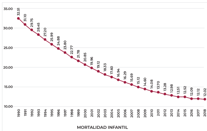
Gráfica 36. México 1990-2018, tasa de mortalidad infantil.
