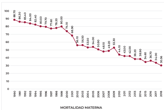
Gráfica 35. México 1990-2018, razón de mortalidad materna.
